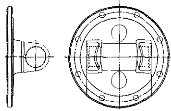
FLANGE YOE
