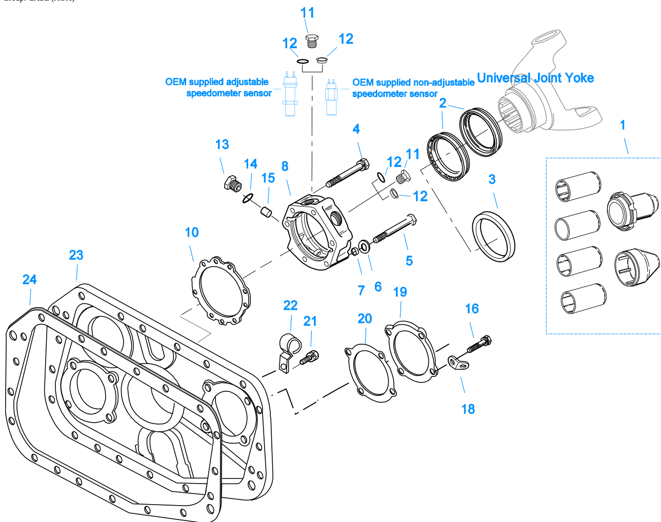
10408-5-94 Aux Case
